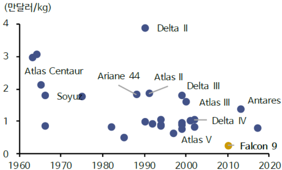
중형급 로켓 발사 비용 추이
